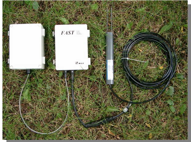
〈写真左より外部電源BOX, FAST-IT本体, TRIME-IT〉
